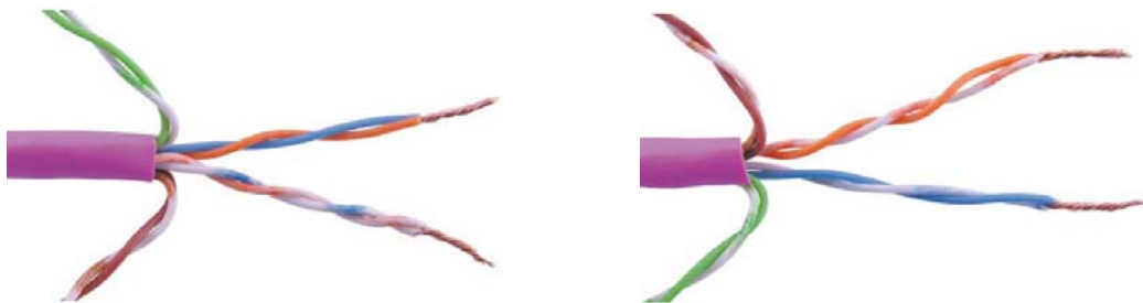
Abbildung 7-3: C-Bus Kabelverwendung Richtig / Falsch [136]
