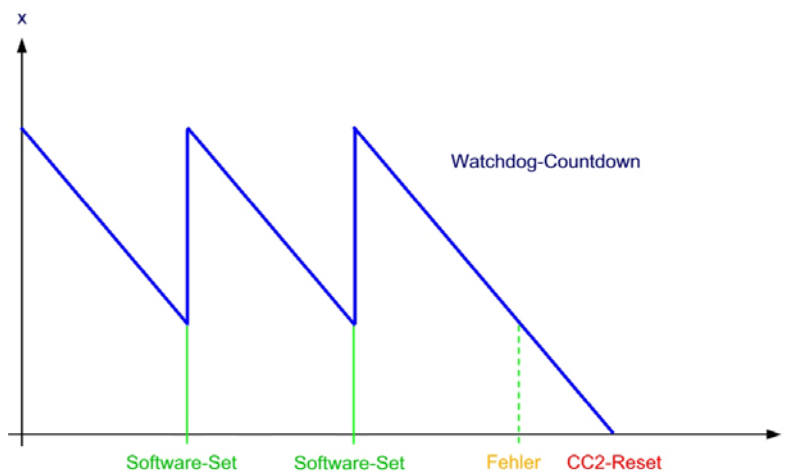
Abbildung 8-9: Praxis-Projekt Watchdog-Timer
