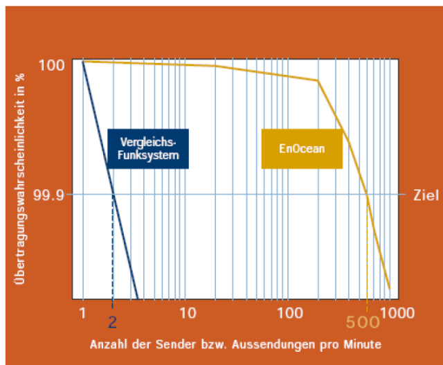
Abbildung 7-2: EnOcean Kollisionssicherheit [132]
