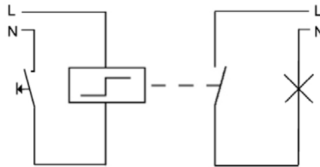
Abbildung 8-5: Praxis-Projekt Stromstoßschalter
