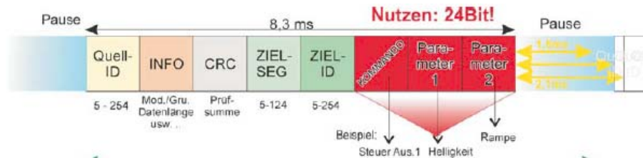
Abbildung 7-9: LCN Datentelegramm [142]
