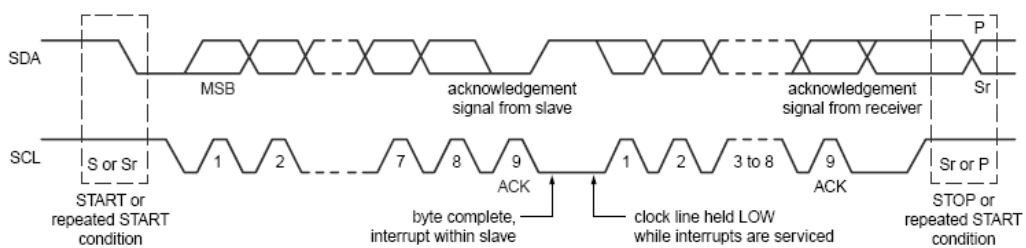
Abbildung 9-5: I 2 C-Bus Datenübertragung ACK/NAK [157]
