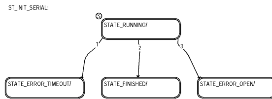
Abbildung 4.4: Initialisierung der seriellen Schnittstelle (Statemachine)
